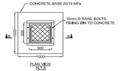
SA STEEL CU-BIN 500x500x900 N.T.S
